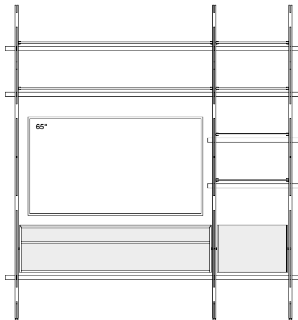
Comp. 309 244,1 x 37 x H 260 cm 3xM2 + 4xR1 + 2xR3 + 1xC2 + 1xC6 tot. 10.860
