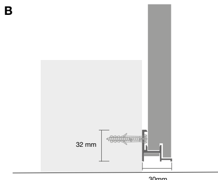
Fissaggio inferiore a parete Lower wall fixing Untere Wandbefestigung Fixation inférieure au mur
