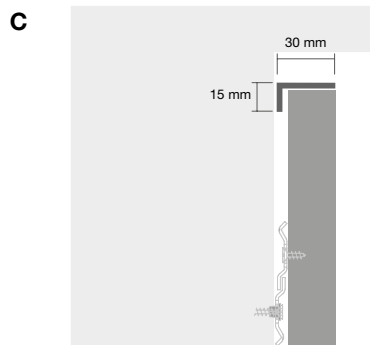
Profilo superiore Upper profile Oberes Profil Profil supérieur
